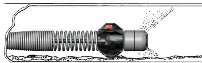
Рисунок 7 – Шаровая направляющая насадка в использовании
