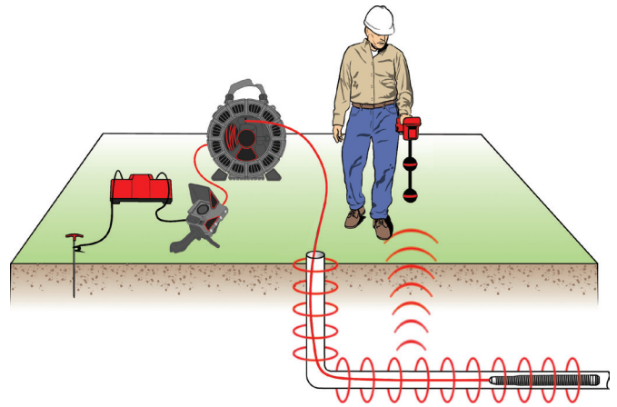
Рисунок 20 – Отслеживание траектории проталкивающего кабеля
